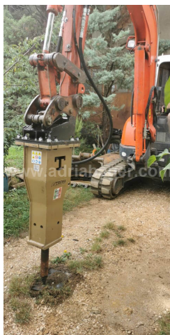
1900 KG, ZA 21-28T BAGER, T1800H HIDRAVLIČNO KLADIVO
