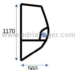
MANITOU MVT, 225234, 746750, 746045, LEVO STRANSKO KALJENO STEKLO
