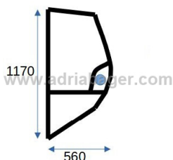
MANITOU MLT, 225234, 746750, 746045, LEVO STRANSKO KALJENO STEKLO
